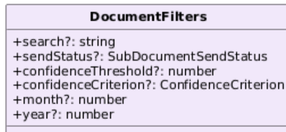
Figura 101: Tipo — DocumentFilters
