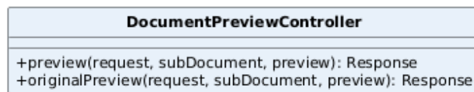
Figura 15: Classe — DocumentPreviewController
