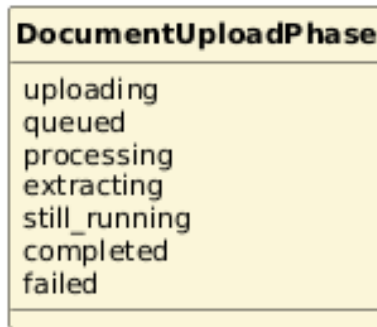
Figura 100: Tipo — DocumentUploadPhase
