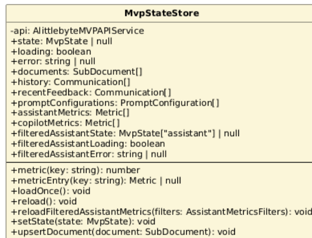
Figura 92: Classe — MvpStateStore
