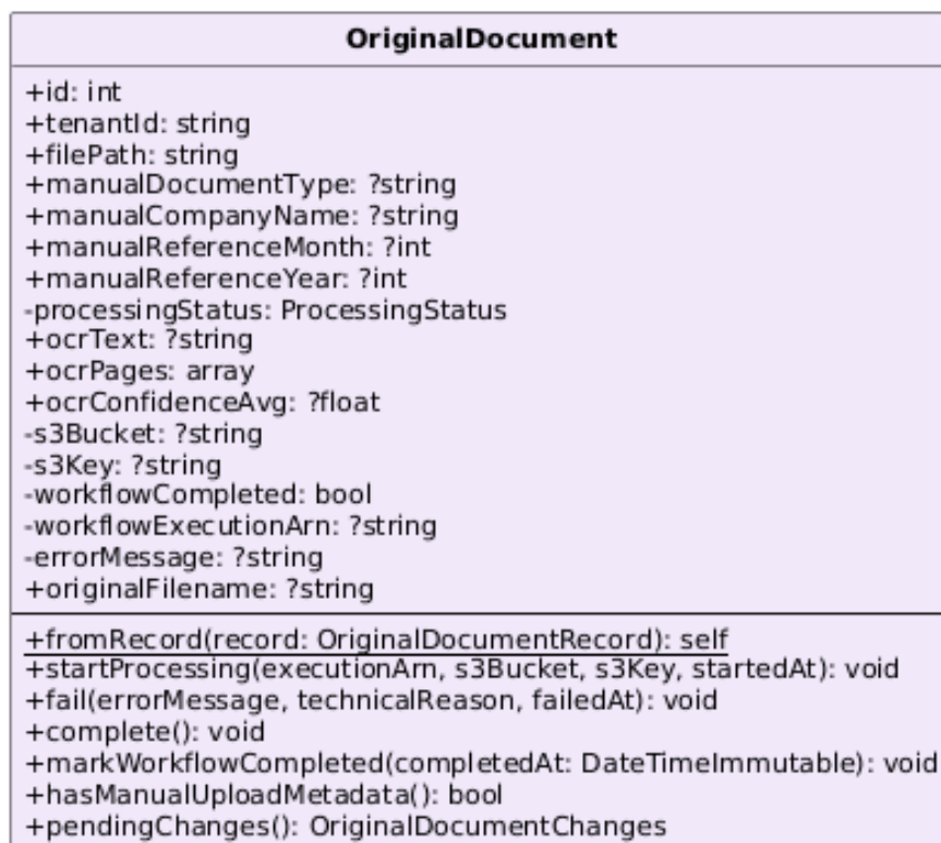
Figura 18: Classe — OriginalDocument
