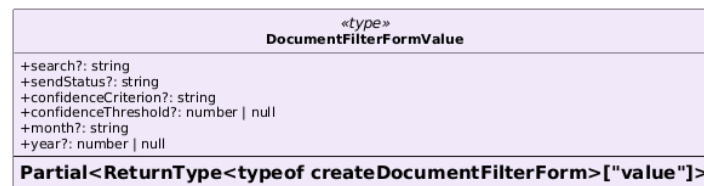
Figura 107: Tipo — DocumentFilterFormValue
