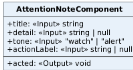
Figura 114: Classe — AttentionNoteComponent
