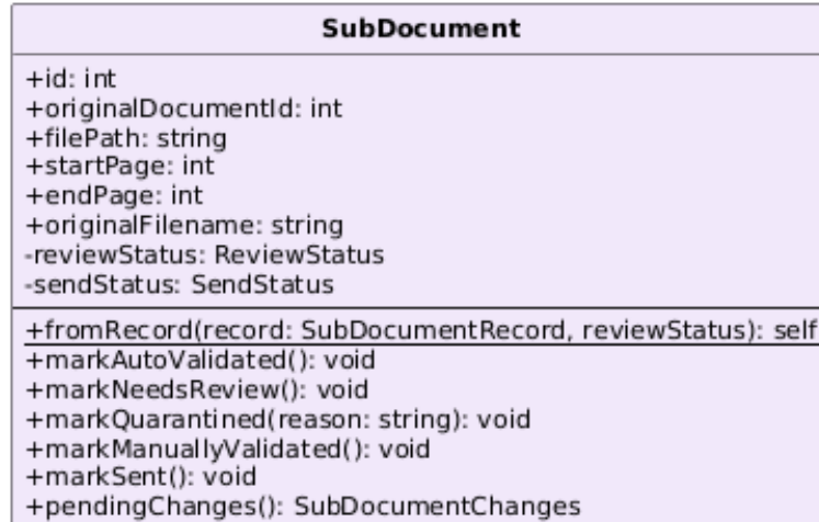
Figura 19: Classe — SubDocument
